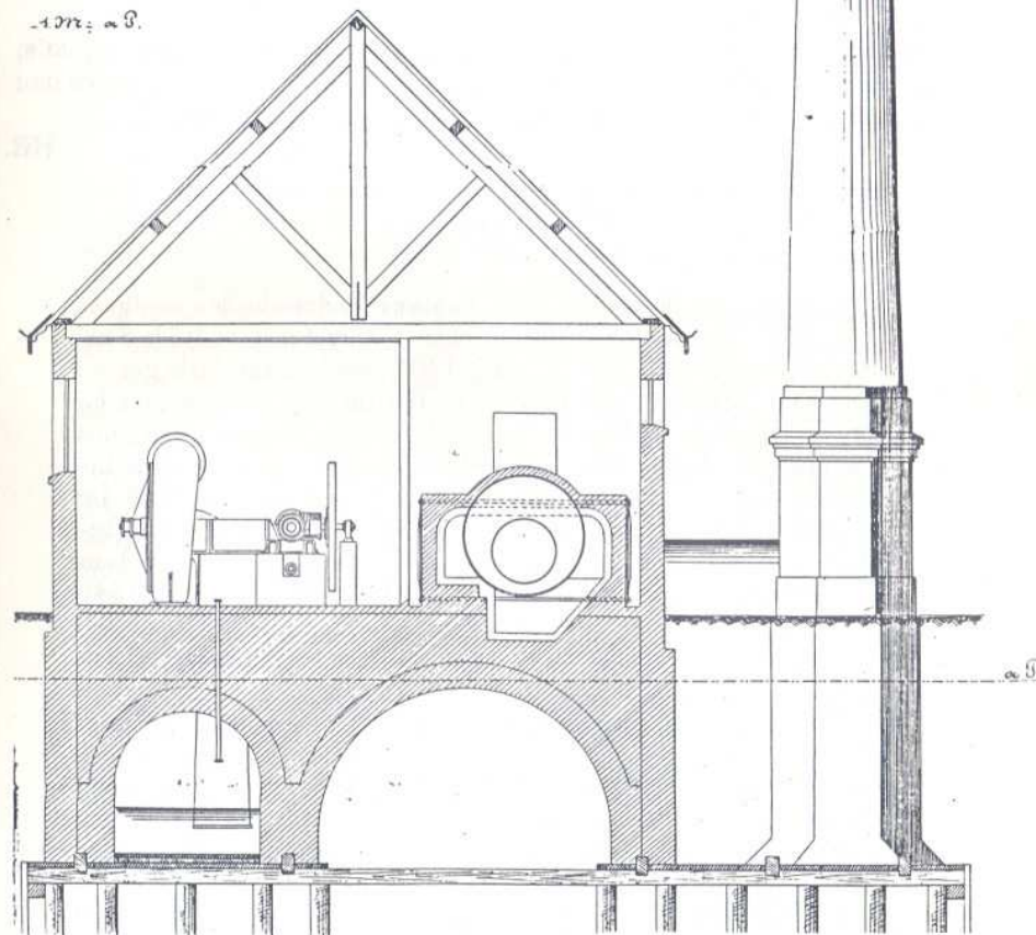
Tekening van het stoomgemaal, gebouwd in 1887.
