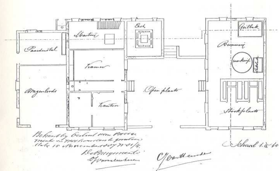
Plattegrond van de bierbrouwerij, waarvoor C.J. van Heusden in 1887 een hinderwetvergunning vroeg.
